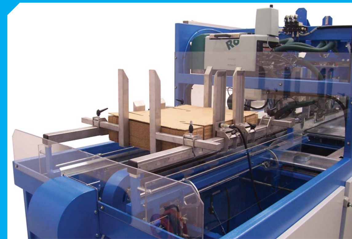
Tray with open columns and front and side double walls Karton mit offenen Ecken zzgl. Doppelwänden an der Längs- und Querseite
